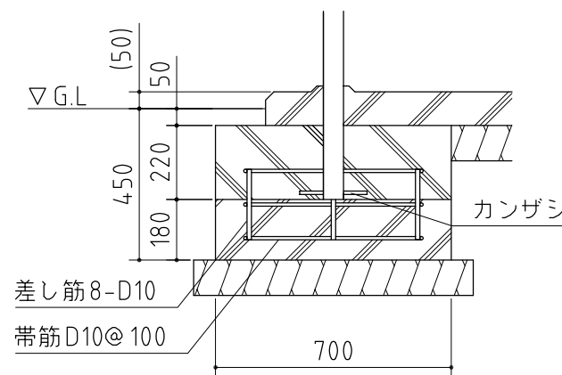
A-A' 断面 1/20
